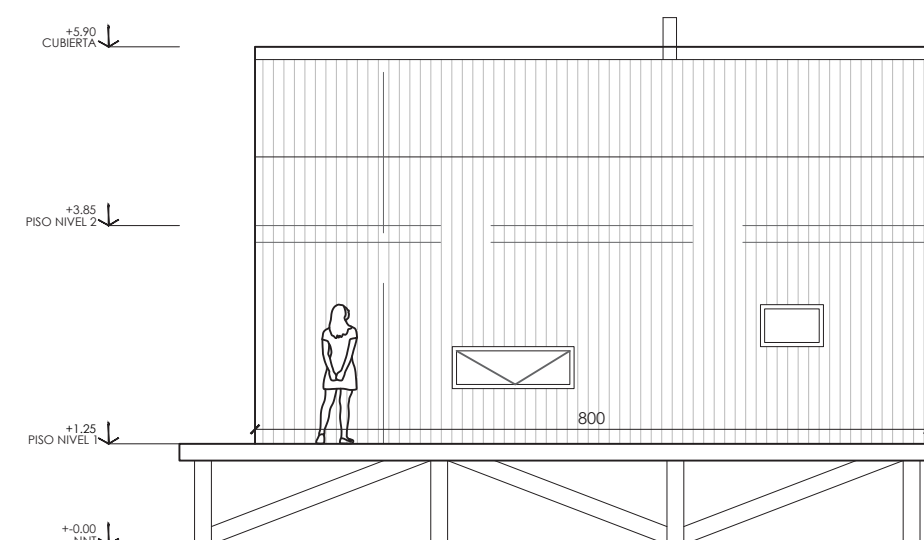
ELEVACION A
