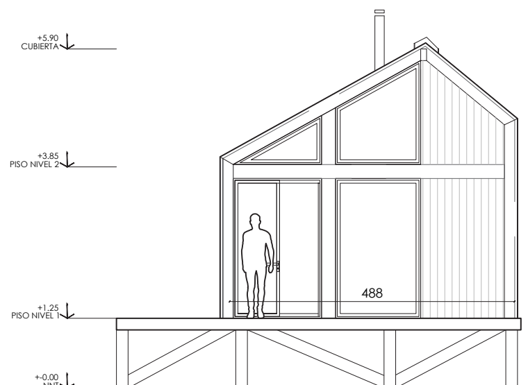
ELEVACION B
